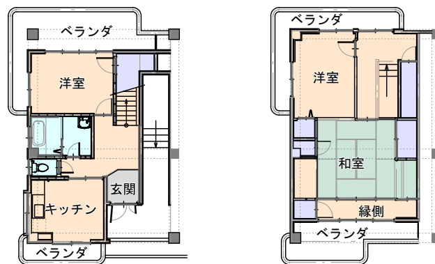
2F平面
